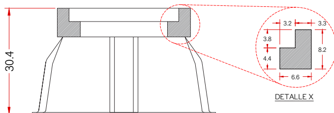
VISTA FRONTAL REGISTRO
