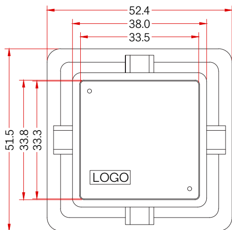
VISTA SUPERIOR REGISTRO
