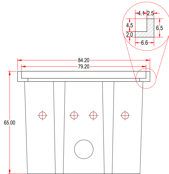
VISTA FRONTAL DEL REGISTRO
