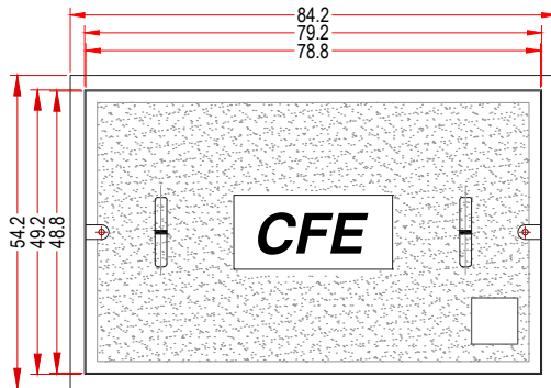
VISTA SUPERIOR DEL MARCO
