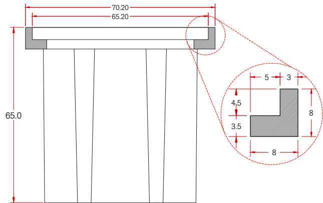
VISTA LATERAL DEL REGISTRO
