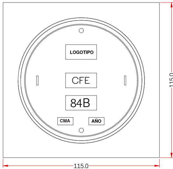
VISTA SUPERIOR DEL REGISTRO
