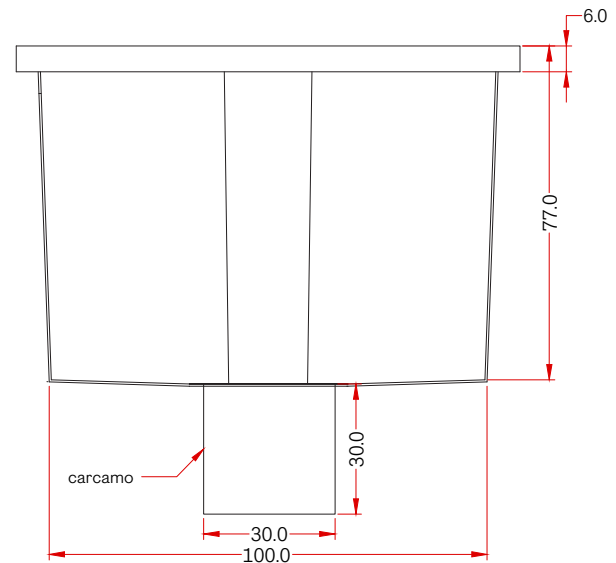
VISTA FRONTAL DEL REGISTRO
